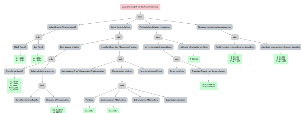
Abb. 5.10: LL5: DoS-Angriff auf das Access Gateway
