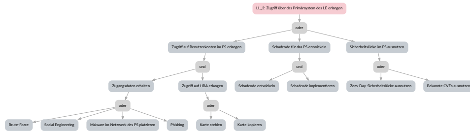
Abb. 5.7: LL2: Zugriff über das Primärsystem des LE erlangen
